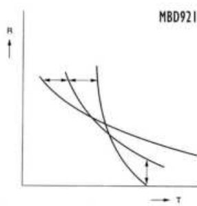
Afb. 2. Het effect van sinteren op de weerstandswaarde als functie van de temperatuur.
